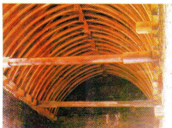
LA CHARPENTE, IDENTIQUE A L'ANCIENNE CHARPENTE DISPARUE
