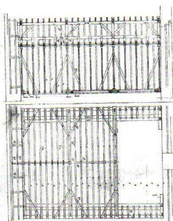
PLAN ET ELEVATION DE LA CHARPENTE SUR LA NEF (COPIE IDENTIQUE DE LA CHARPENTE DE 1545)
