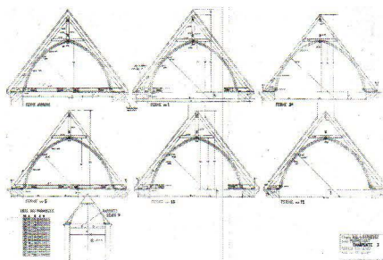
LES PRIMES SUR LA NEF
