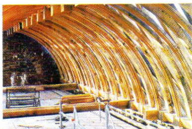
PENDANT LA POSE DE LA CHARPENTE
