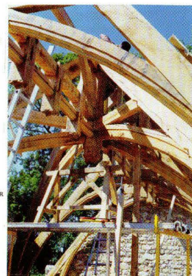
LA CHARPENTE SUR LE CHOEUR
