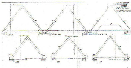
RELEVÉS DES PIGNONS INTÉRIEURS
