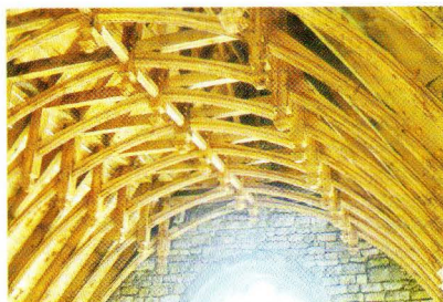
LA CHARPENTE EN CHÊNE AVEC POINÇONS, ENGOULANTS, ET CORNICHES SCULPTÉES
