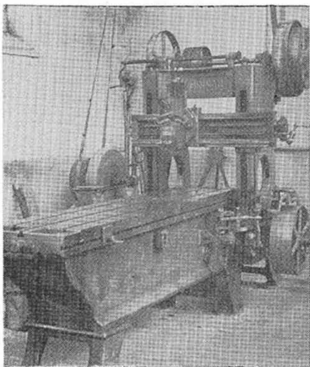
Raboteuse « Cincinnati »
