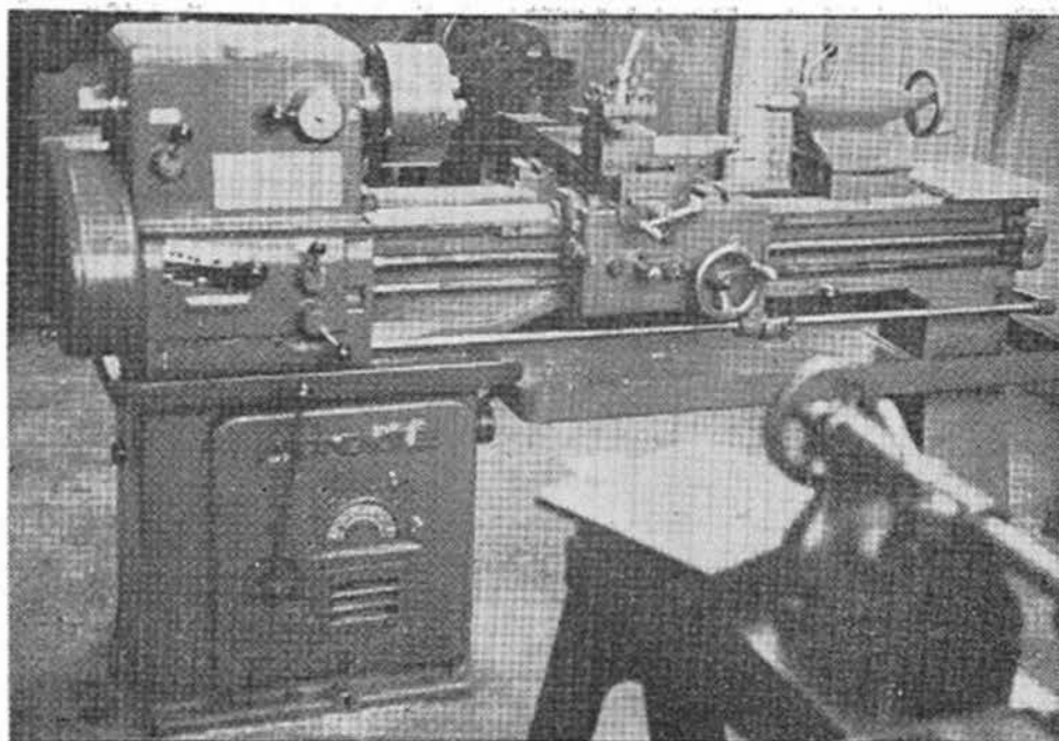
Tour « Mondiale »
