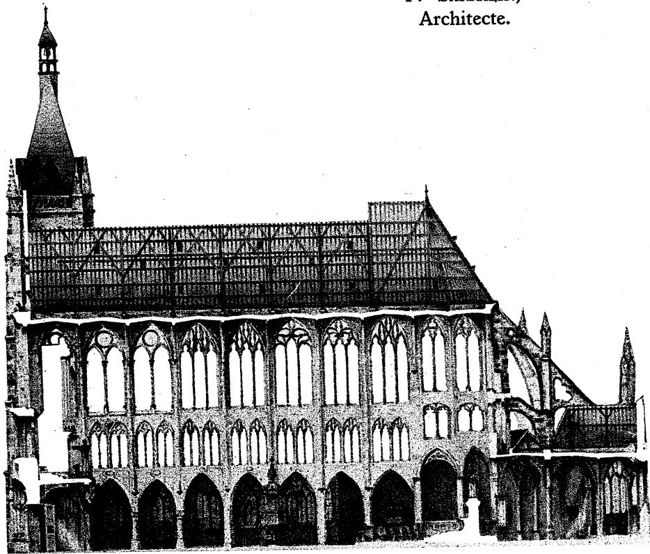
FAÇADE PRINCIPALE ET COUPE LONGITUDINALE DE L'ÉGLISE SAINT-SÉVERIN. (Dessins dressés et exécutés à la plume par P. Sarrazin.)
