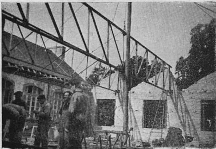
Montage de la charpente des ateliers
