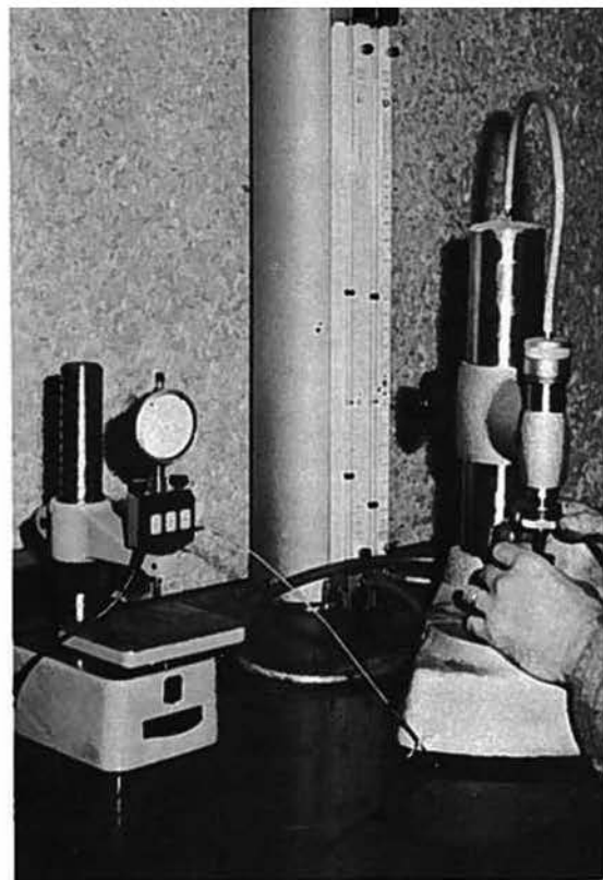
Comparateur pneumatique « Solex »
