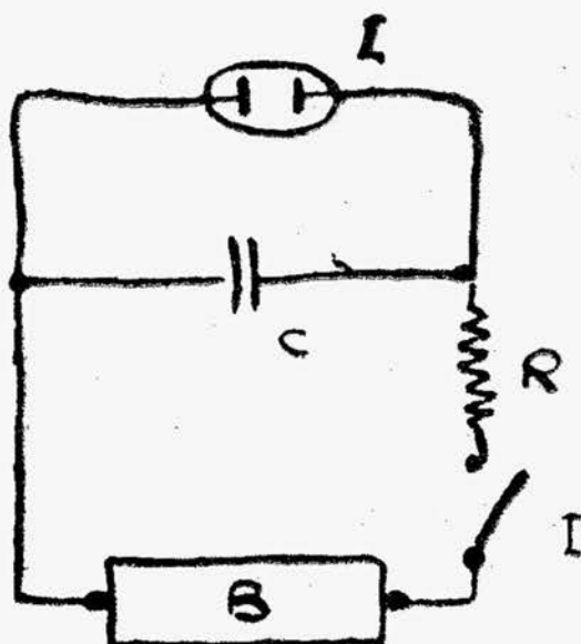
Accumulateur à l'iode.
