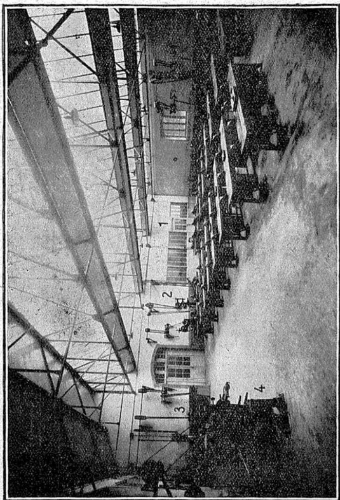
1. Vitrage sur les forges. — 2. Scies à métaux. — 3. Perceuses, meules diverses. — 4. Rangée de moteurs, fraiseuse.
