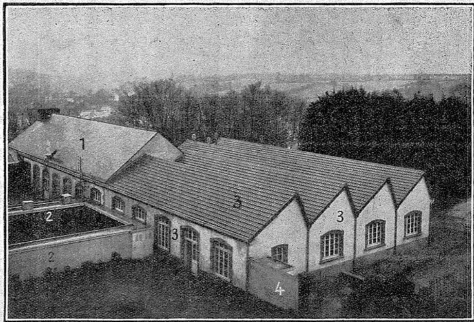
1. Anciens ateliers (ajustage, forge et tours), aujourd'hui ateliers à bois. Salle de modelage. Vestiaire et lavabos. 2. Nouveaux W.-C. — 3. Nouveaux ateliers (forges, étaux, tours, moteurs divers. — 4. Entrée du jardin.
